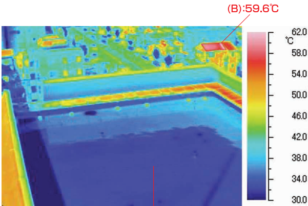
■左写真のサーモグラフィによる画像
